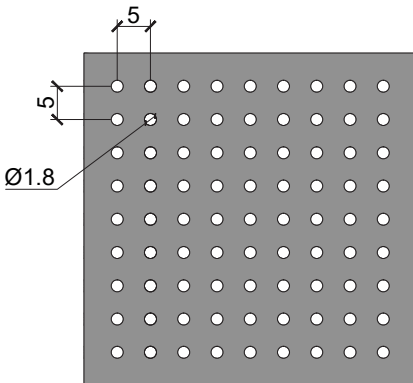
Perforasyon / Perforation Boşluk Oranı / Open Area Ø1,8 mm %10,20
