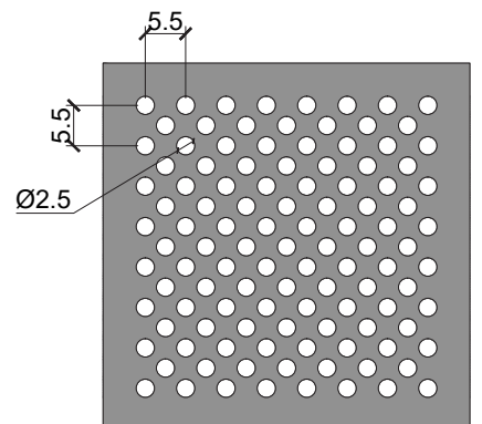
Perforasyon / Perforation Boşluk Oranı / Open Area Ø2,5 mm %32,10
