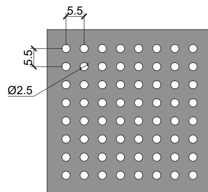
Perforasyon / Perforation Boşluk Oranı / Open Area Ø2,5 mm %16,20
