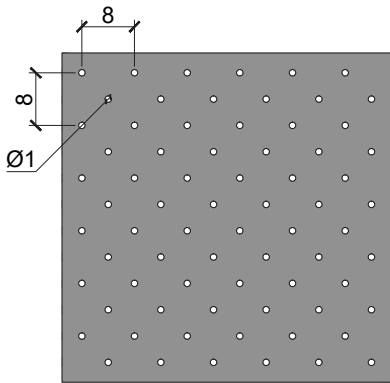
Perforasyon / Perforation Boşluk Oranı / Open Area Ø1,5 mm %2,46
