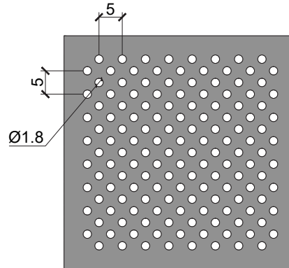
Perforasyon / Perforation Boşluk Oranı / Open Area Ø1,8 mm %20,30
