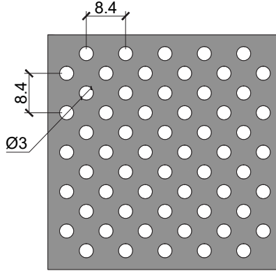
Perforasyon / Perforation Boşluk Oranı / Open Area Ø3 mm %20
