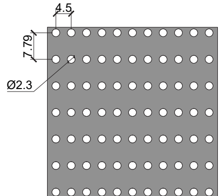
Perforasyon / Perforation Boşluk Oranı / Open Area Ø2,3 mm %11,80
