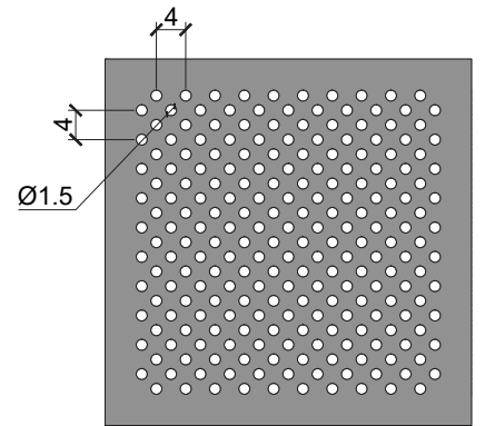
Perforasyon / Perforation Boşluk Oranı / Open Area Ø1,5 mm %22
