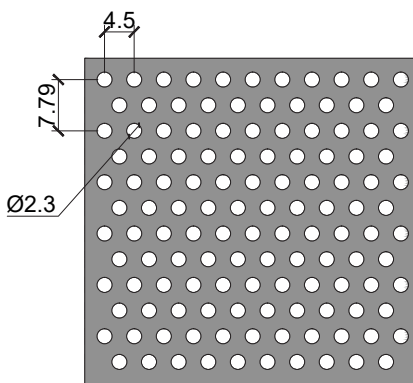
Perforasyon / Perforation Boşluk Oranı / Open Area Ø2,3 mm %23,69
